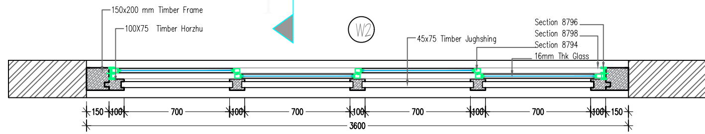
SECTION a-a
